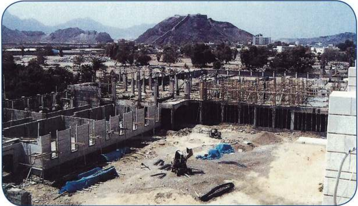
مشروع بناء كلية الصيدلة بجامعة عدن في الجمهورية اليمنية: مبنى الكلية، وقد توسطت أعمال بناء الدور الأول في ٢٠٠٧/٢/١٩
